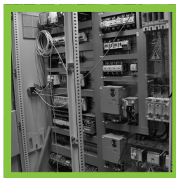
Câblage
