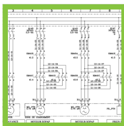
Etudes électriques
