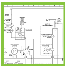
Etudes hydrauliques
